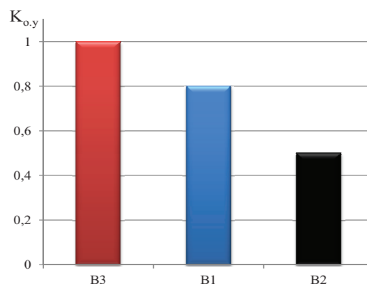
Рис. 5. Относительный коэффициент износостойкости образцов исходных материалов к абразиву № 5
