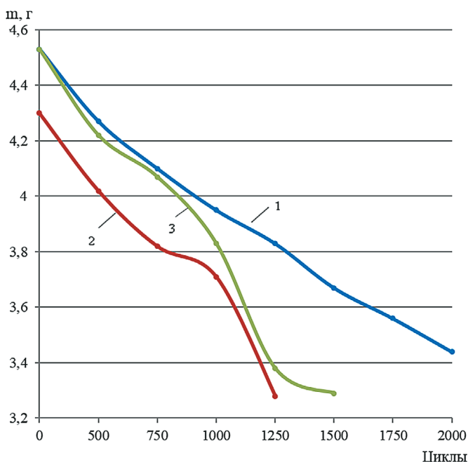
Рис. 1. Изменение массы войлока технического B_1 при истирании:
