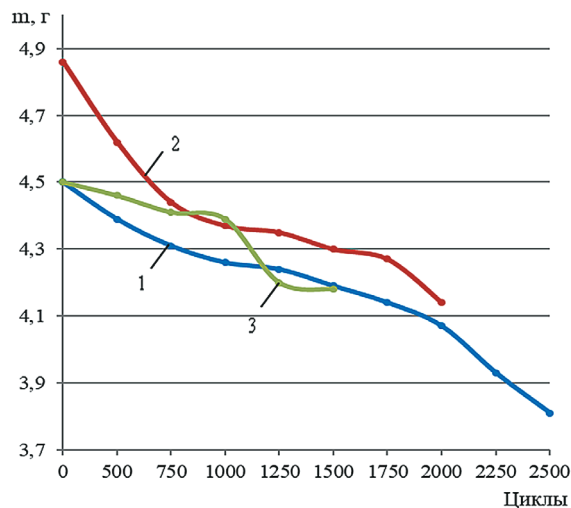
Рис. 3. Изменение массы войлока обувного В 3 при истирании:
