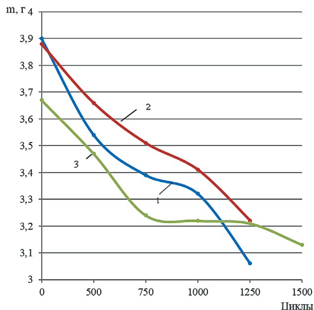
Рис. 2. Изменение массы войлока технического B_2 при истирании:
