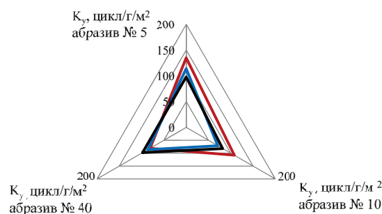
Рис. 4. Коэффициент устойчивости к истиранию исходных материалов: ■ – B 1 , ■ – B 2 , ■ – B 3
